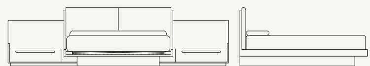
BRO TAPIZADO mesita: 50 - 60 - 70 - 80 aro: 135 - 150 - 160 - 180 x 190 - 200 alto: 90
