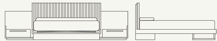
BRO VERTICAL mesita: 50 - 60 - 70 - 80 aro: 135 - 150 - 160 - 180 x 190 - 200 alto: 90
