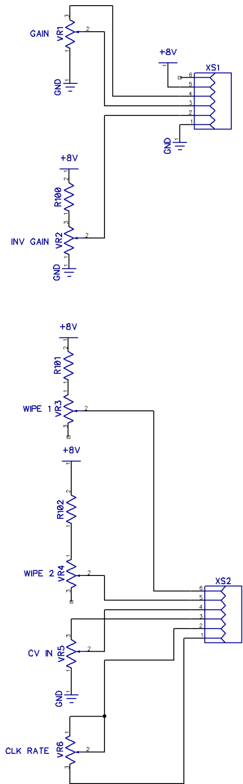
TRQ V2 Control Board - Syntonie 2018
